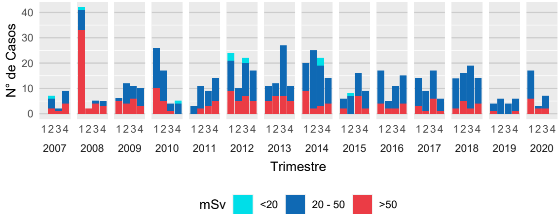
Figura 2: Distribución de Alertas de Cuerpo Entero por rango de Proyección de dosis anual, por año y trimestre. Chile, 2007 – 2020*
